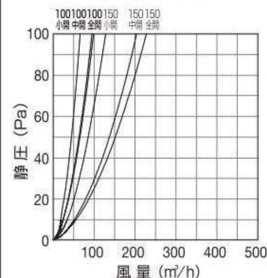
圧力損失曲線
