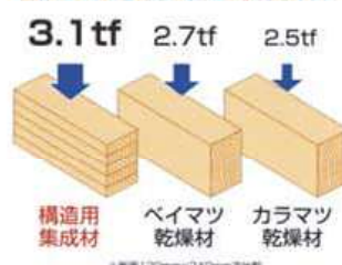
梁・桁材の長期許容曲げ応力比較
