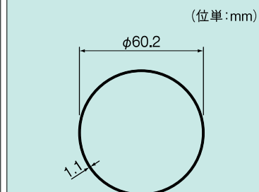
たてどい(60)断面図
