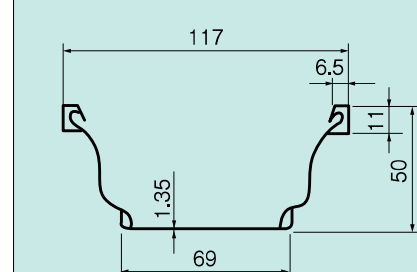
軒どい(117)断面図(位単:mm)
